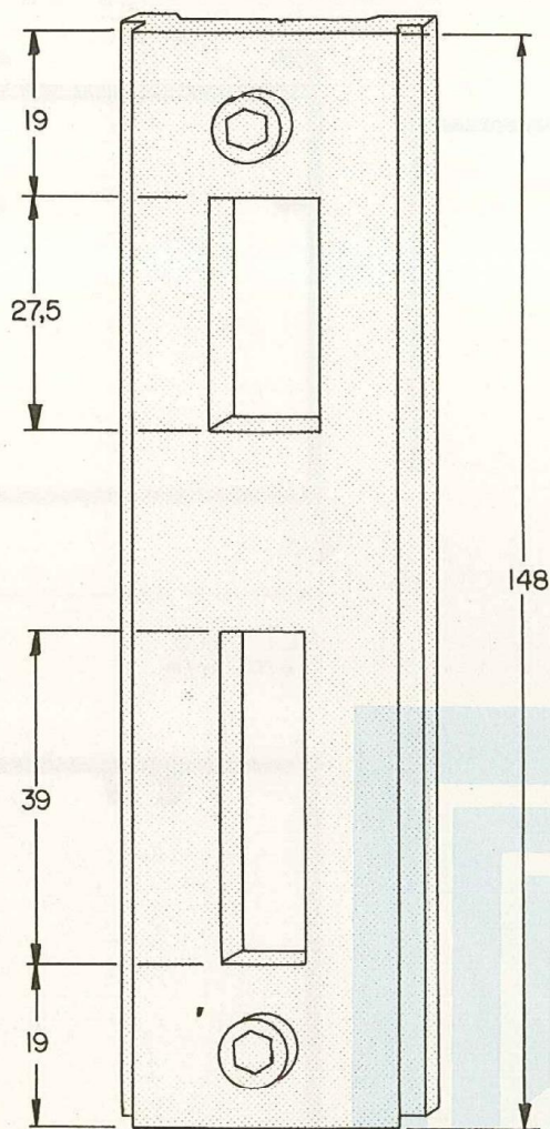
CONTRATESTA ALUMÍNIO
