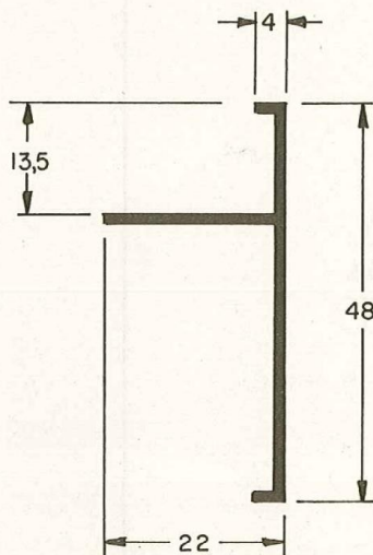
ALS 591 0,300 Kg/m
