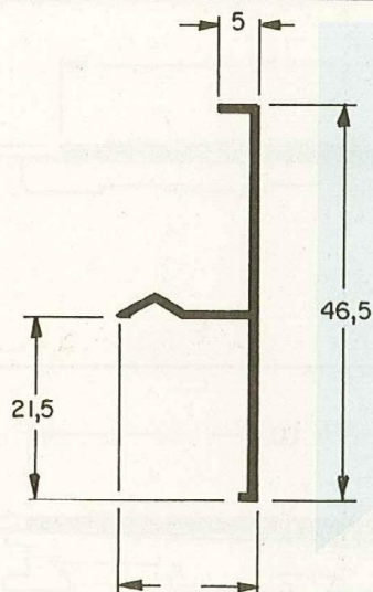
ALS 509 0,185 Kg/m
