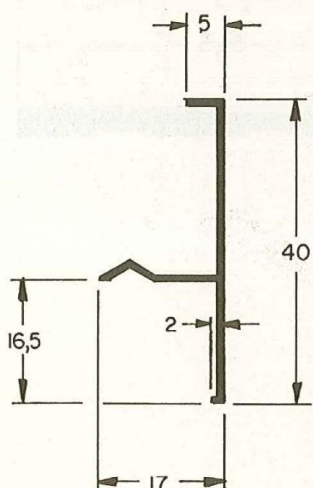
ALS 509 0,185 Kg/m
