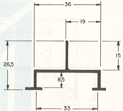
ALS 504 0,301 Kg/m
