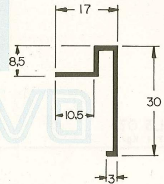
ALS 042 0,179 Kg/m
