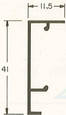
ALS 002 0,658 Kg/m
