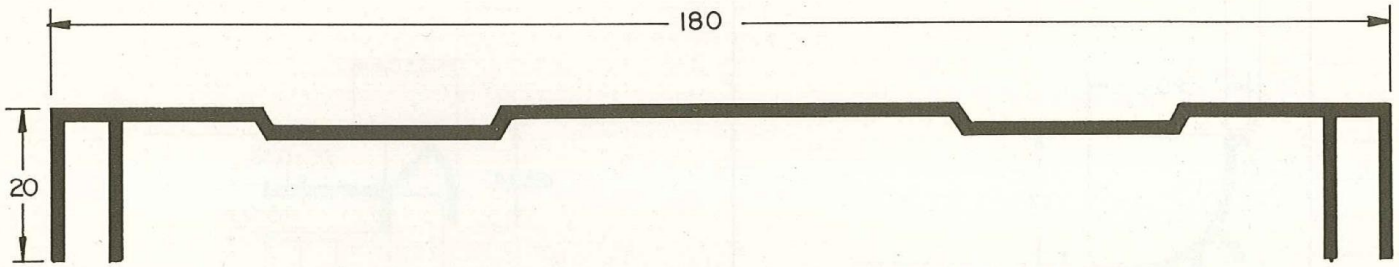
ALS 574 1,393 Kg/m
