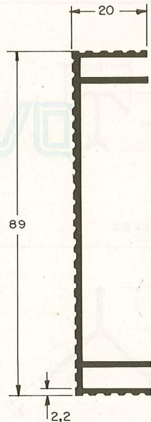
ALS 572 0,635 Kg/m
