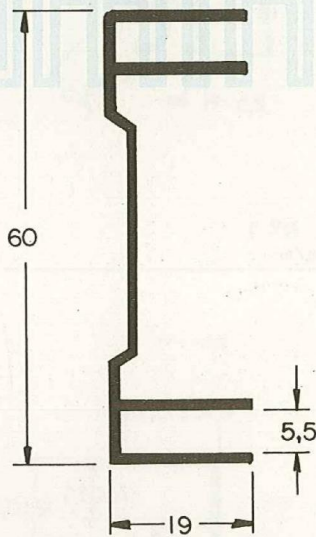
ALS 570 0,534 Kg/m
