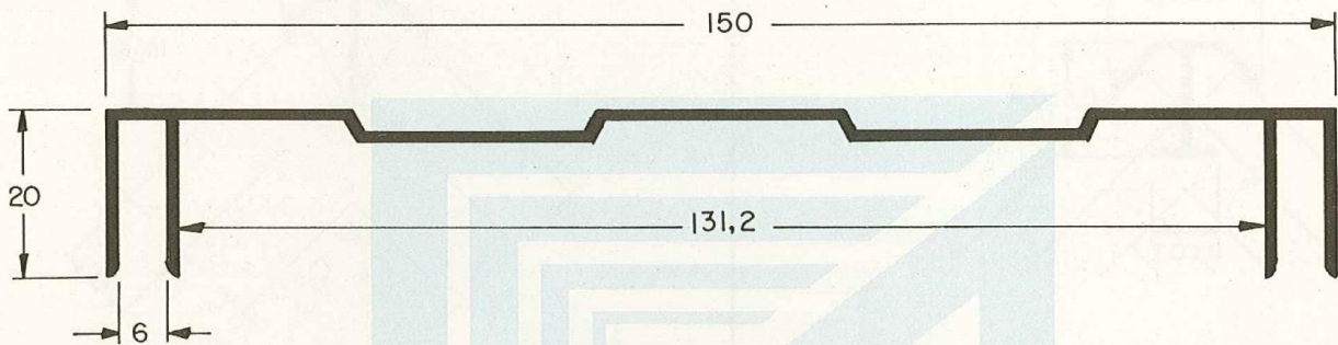
ALS 573 1,050 Kg/m
