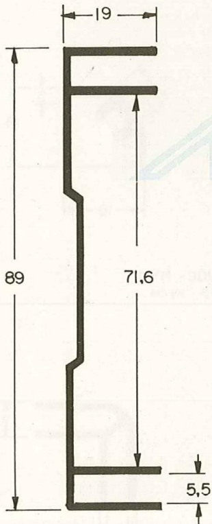
ALS 571 0,650 Kg/m
