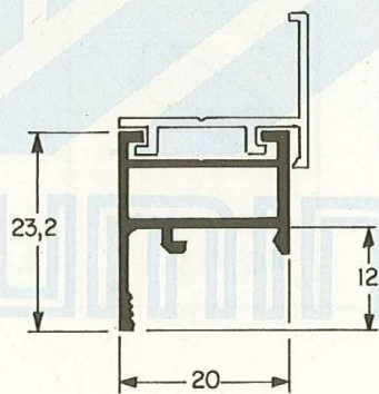
ALT 117 0,280 Kg/m
