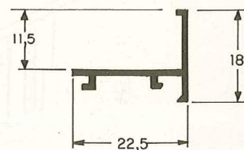
ALS 120 0,176 Kg/m
