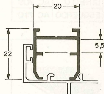
ALS 115 0,270 Kg/m
