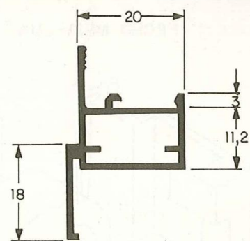
ALT 112 0,360 Kg/m
