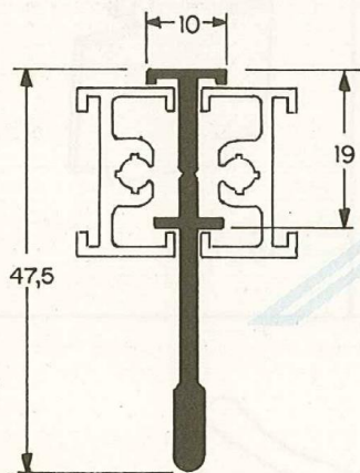
ALS 116 0,415 Kg/m
