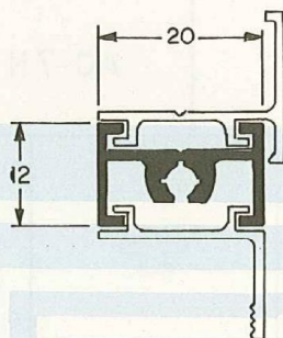
ALS 114 0,220 Kg/m
