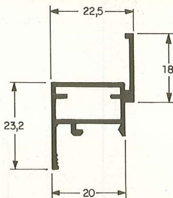
ALT 111 0,360 Kg/m
