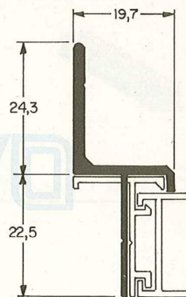
ALS 118 0,360 Kg/m
