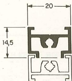
ALS 113 0,245 Kg/m
