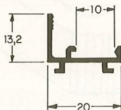
ALS 119 0,165 Kg/m
