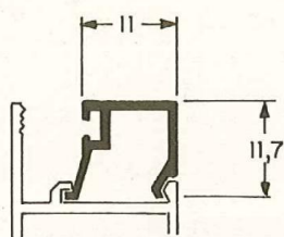
ALS 264 0,100 Kg/m
