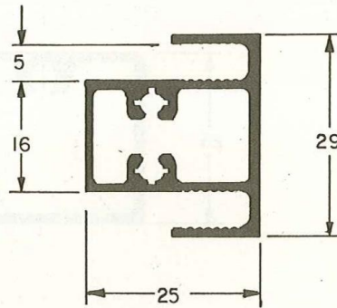
ALT 280 0,569 Kg/m
