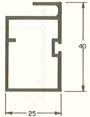
ALT 277 0,580 Kg/m
