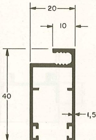
ALS 503 0,490 Kg/m
