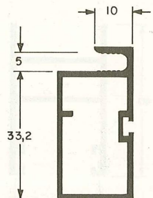
ALT 502 0,525 Kg/m
