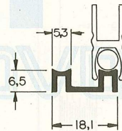
ALS 618 0,155 Kg/m
