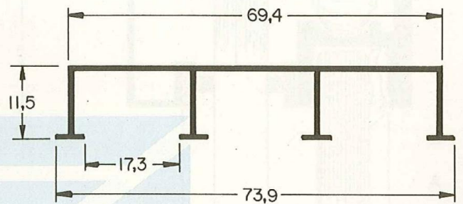
ALS 545 0,293 Kg/m
