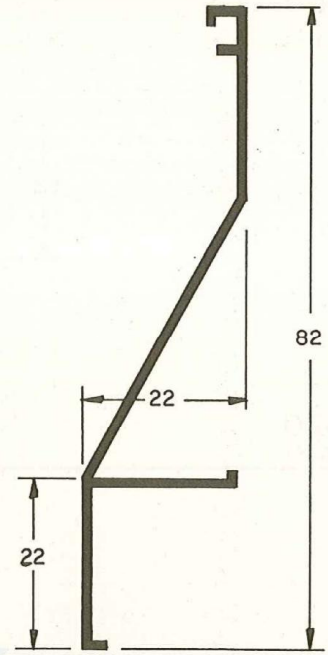
ALS 535 0,424 Kg/m
